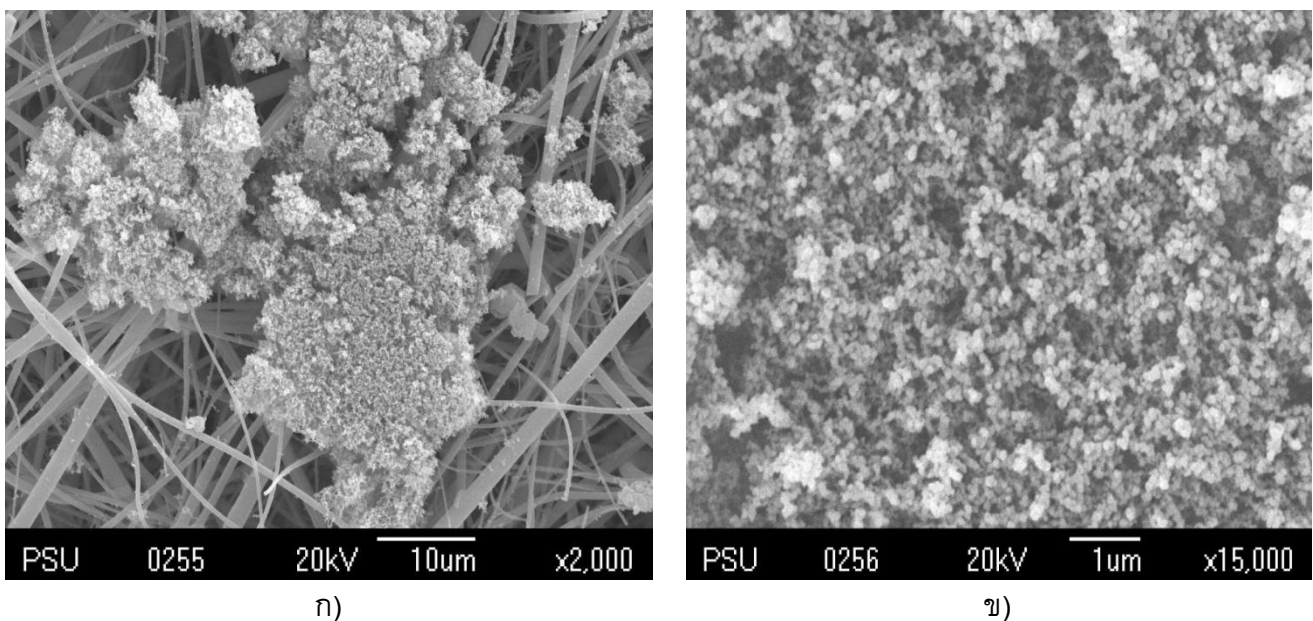
ภาพที่ 4.3 ภาพถ่ายฝุ่นละอองบนกระดาษกรองที่เก็บได้ด้วยเครื่อง SEM
