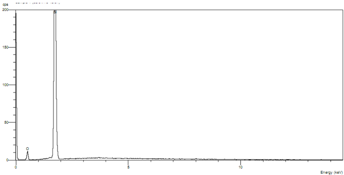
ภาพที่ 4.2 ลักษณะสเปกตรัมของกระดาษกรองใยแก้ว
